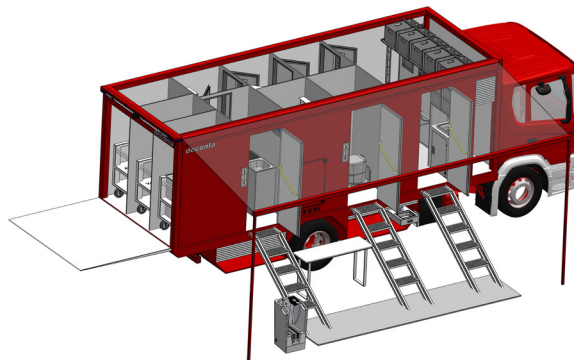
FAHRZEUGAUFBAU
